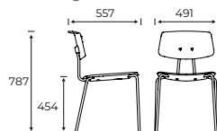
Share Basic, Rückenlehne Polypropylen, mit Sitzpol- sterung
