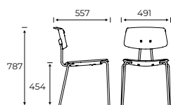
Share Basic, Rückenlehne Poly- propylen, Sitzfläche Eiche Natur, ohne Polsterung
